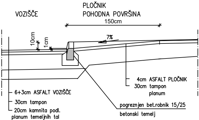
Prerez A-A M 1:50
